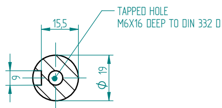
Przekrój A-A 1:1
